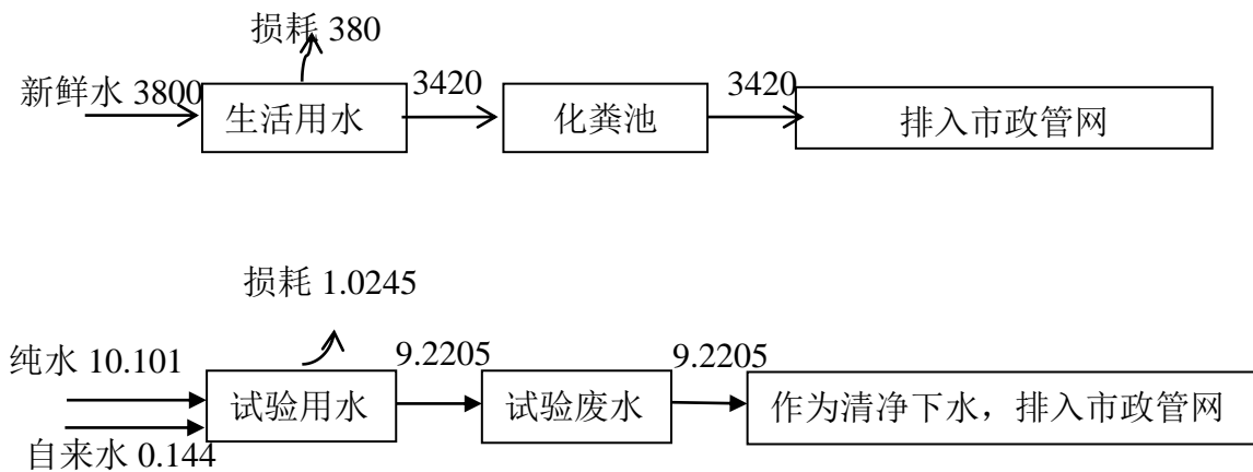
图 2-1 项目水平衡图 (单位: m³/a)
