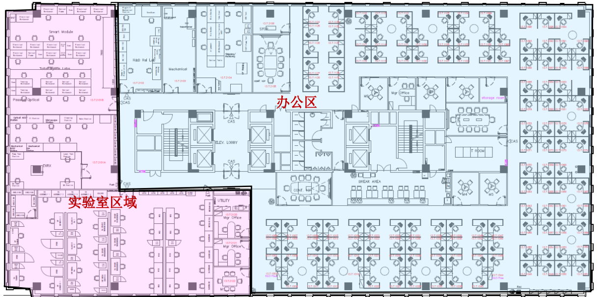
项目 7 层平面布置图:
